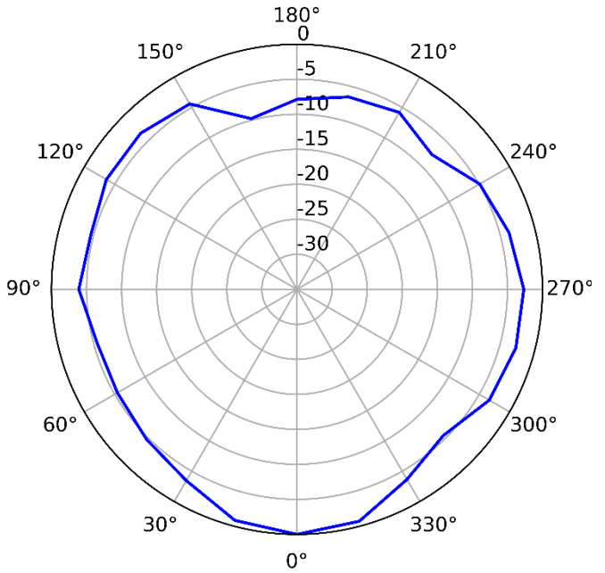
2.4 GHz (vertical)
